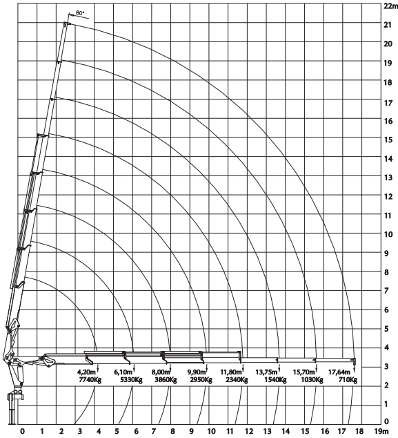
Gráfico de Carga | Gráfico de carga
