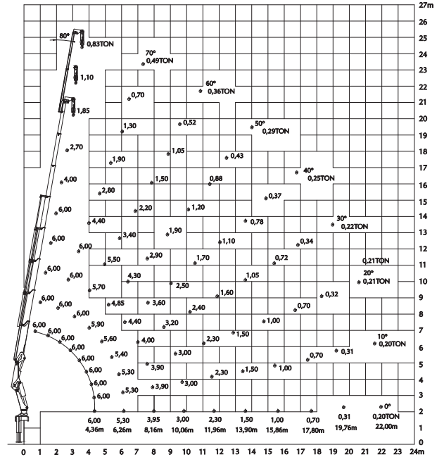
Gráfico de Carga com Guincho e lança JIB | Gráfico de Carga con Guinche y Plumín
