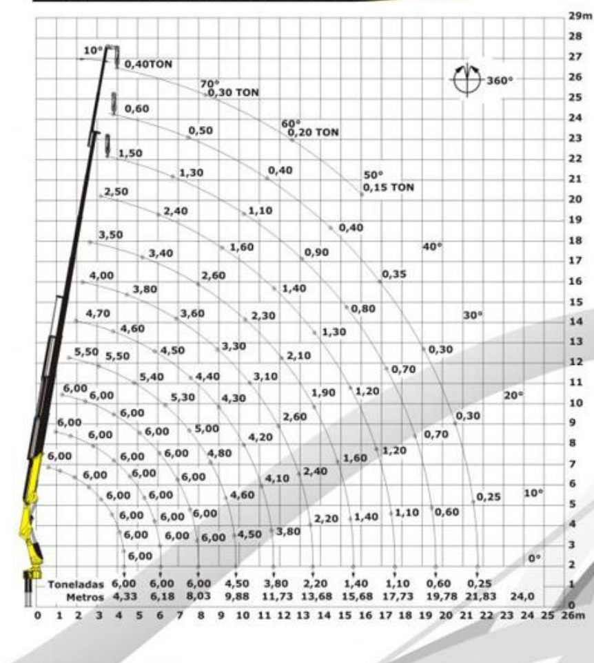
Gráfico de Carga com Guincho e Jib
