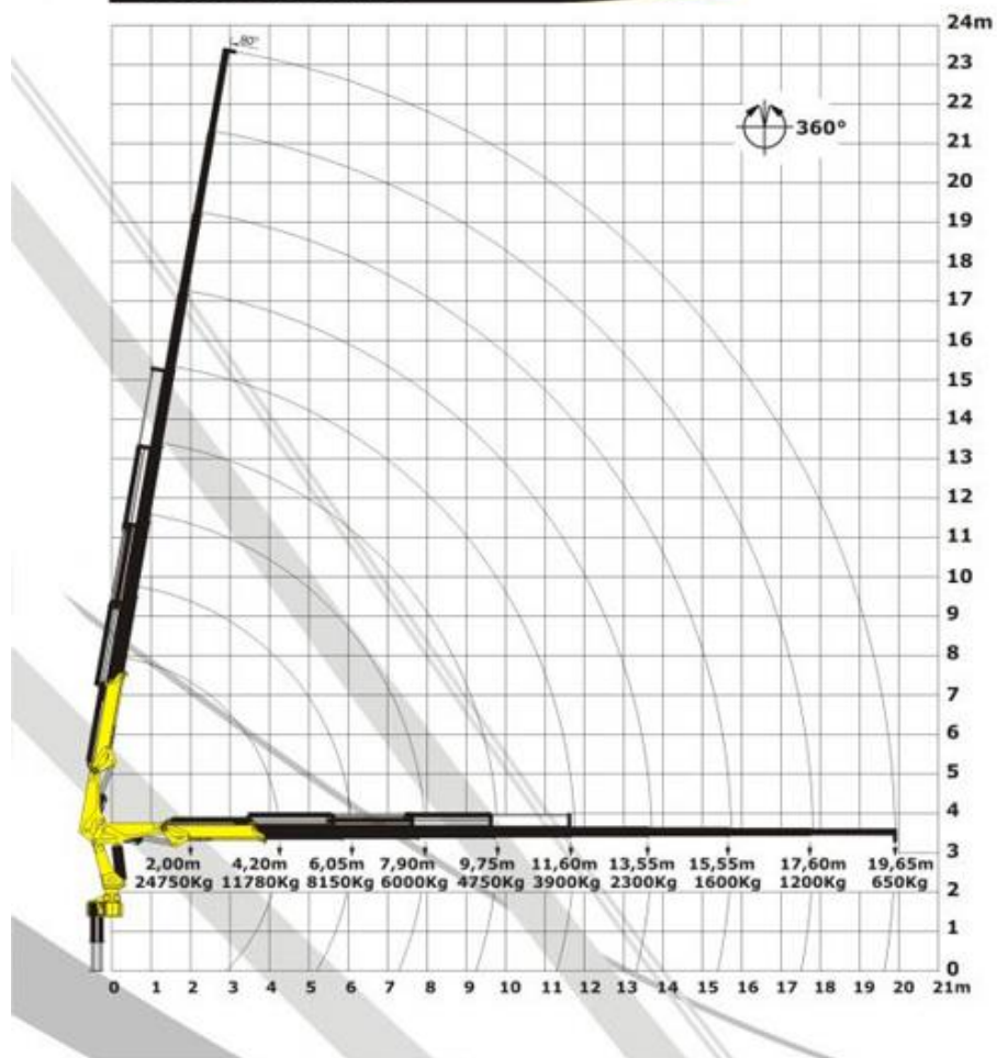
Gráfico de Carga
